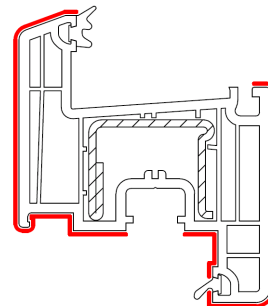
anta Z60
