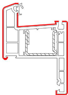
telaio 60/40
