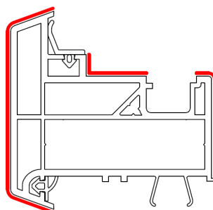
scambio battuta
